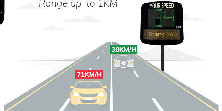
RAD60
